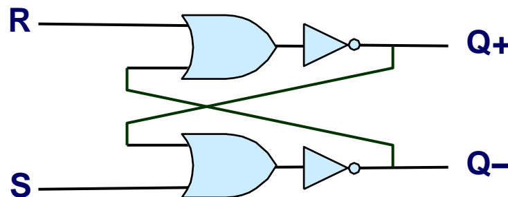
R-S锁存器 R-S Latch
